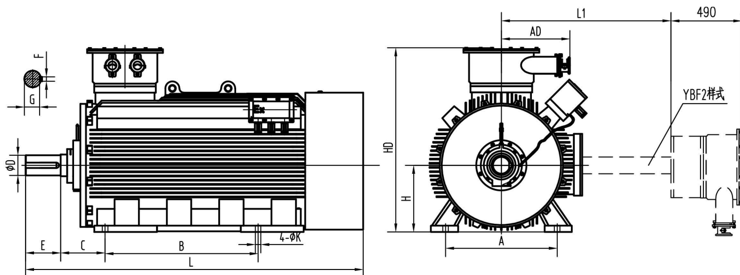
YBX3高效率隔爆型三相异步电动机外形安装尺寸及公差
