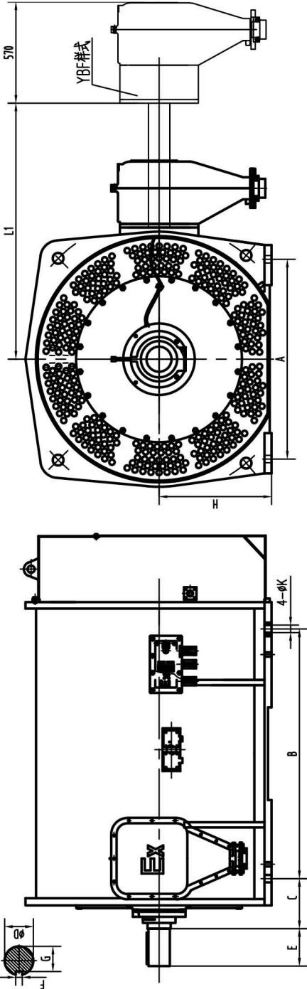
YB高压隔爆型三相异步电动机H560-800
